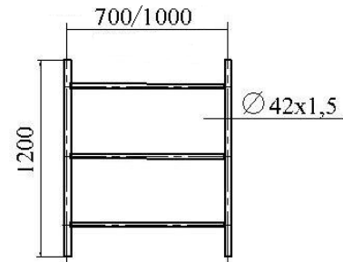
стяжка ограждения (8)
