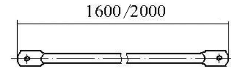
перекладина ограждения (9)
