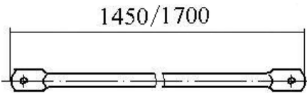
стяжка рядовая (5)
