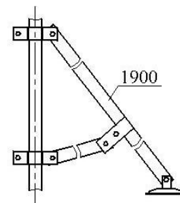
опора-стабилизатор (12)
